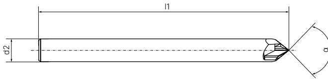
α Spitzenwinkel point angle
